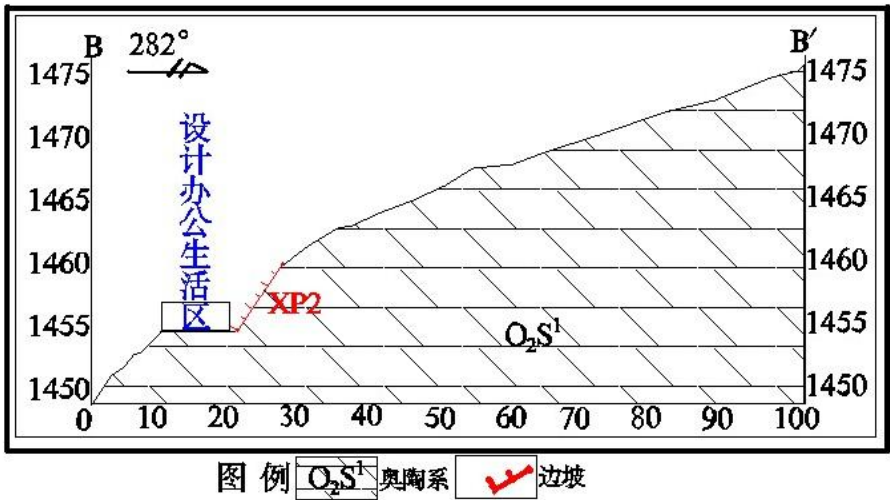
图 8-3-2XP2 剖面图
