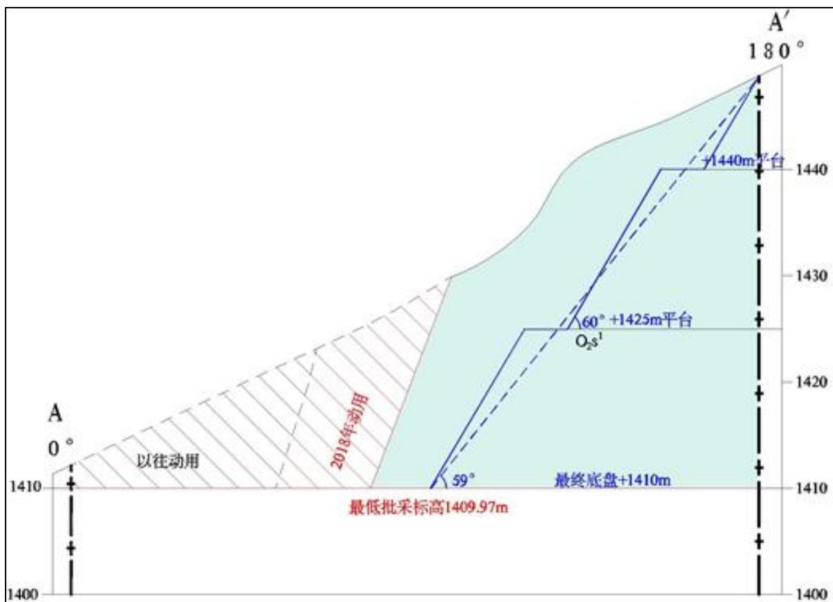
图 8-3-1 终了边坡示意图
