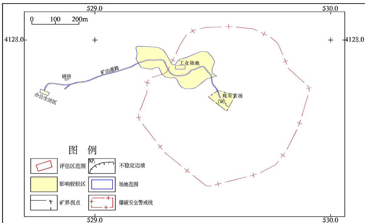
图 8-2-2 采矿活动对含水层影响现状评估分区图
