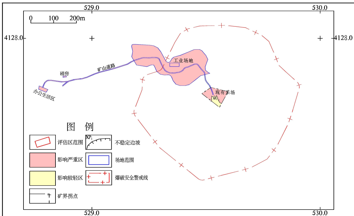
图 8-1-3 采矿活动对地形地貌景观影响现状评估分区图
