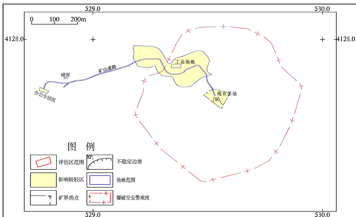
图 8-2-1 地质灾害影响程度现状评估分区图
