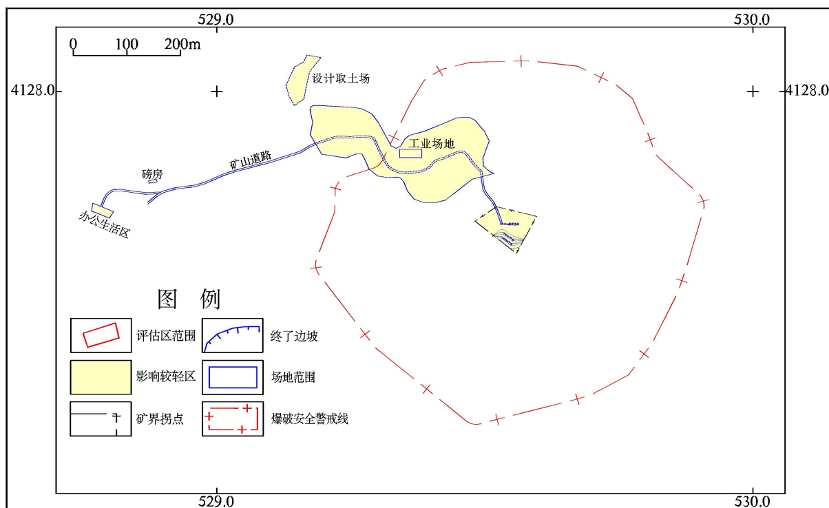
图 8-3-6 服务期采矿活动对含水层影响预测评估分区图
