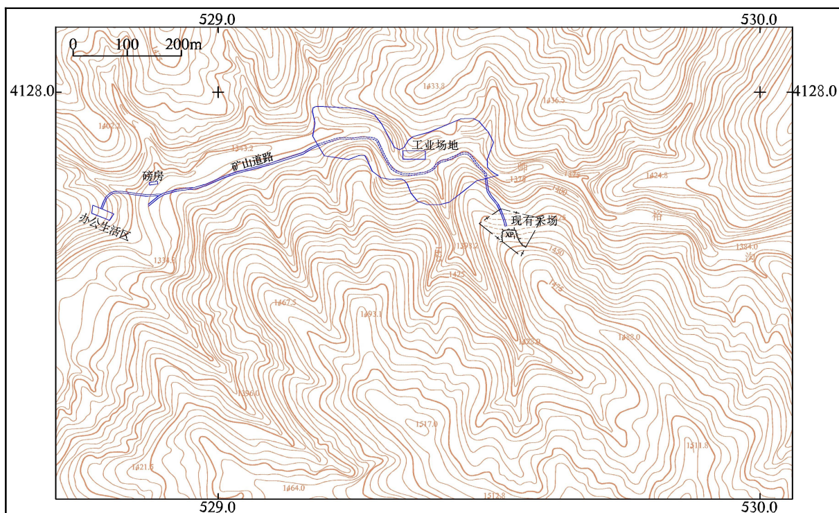
图 8-3-2 师裕沟汇水范围图
