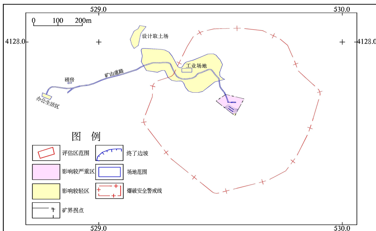
图 8-3-4 服务期地质灾害影响预测评估分区图
