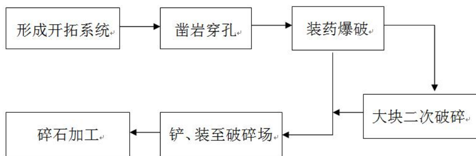
开采工艺图
