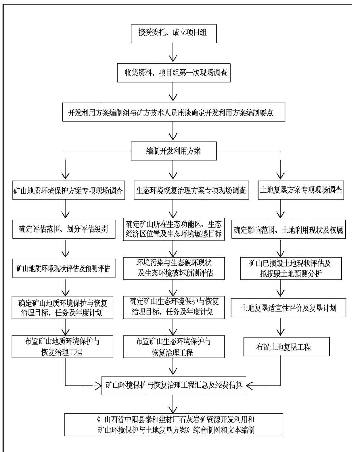
图 1-2 工作流程图
