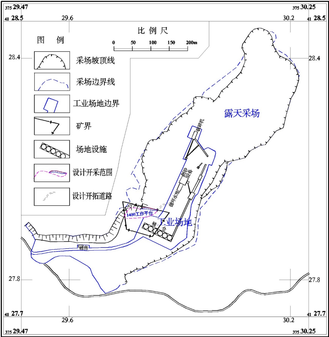
图 5-1 总平面布置图
