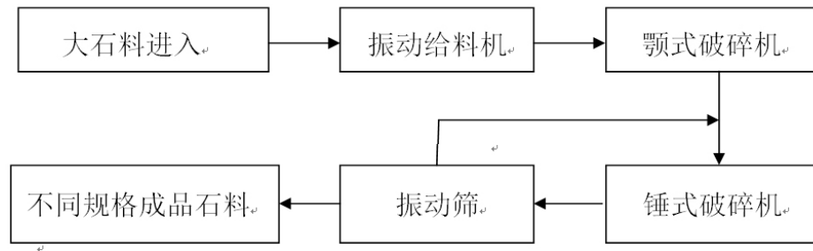
图 5-3 生产线流程图
