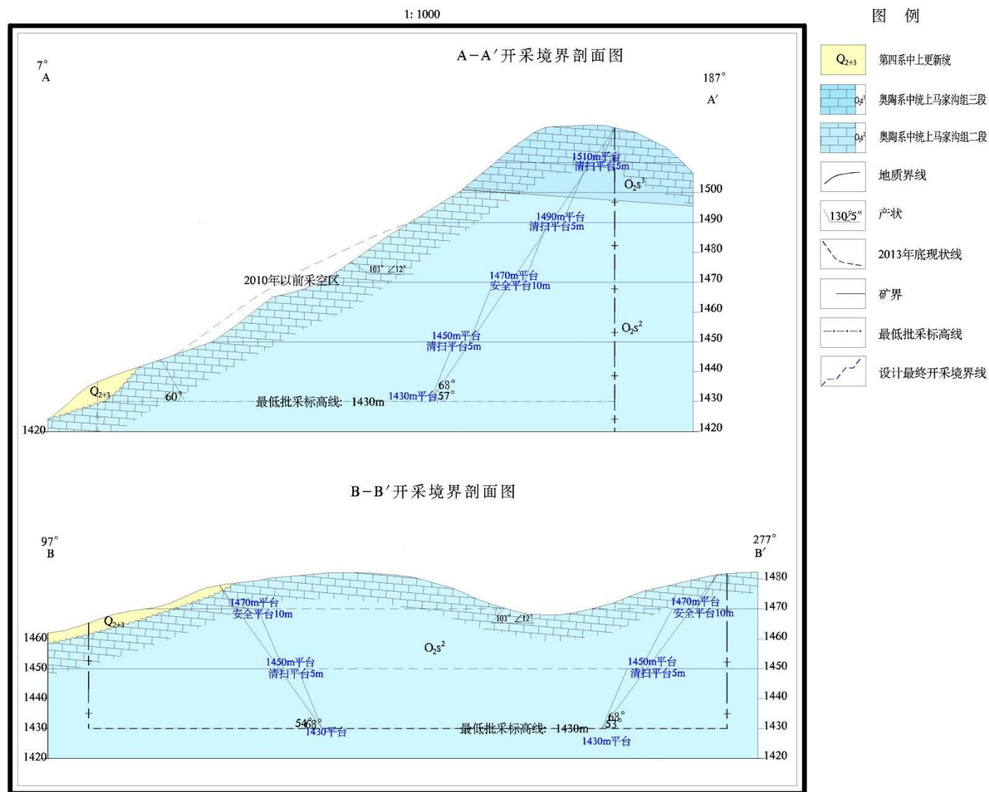
图 8-3-1 采掘终了剖面图
