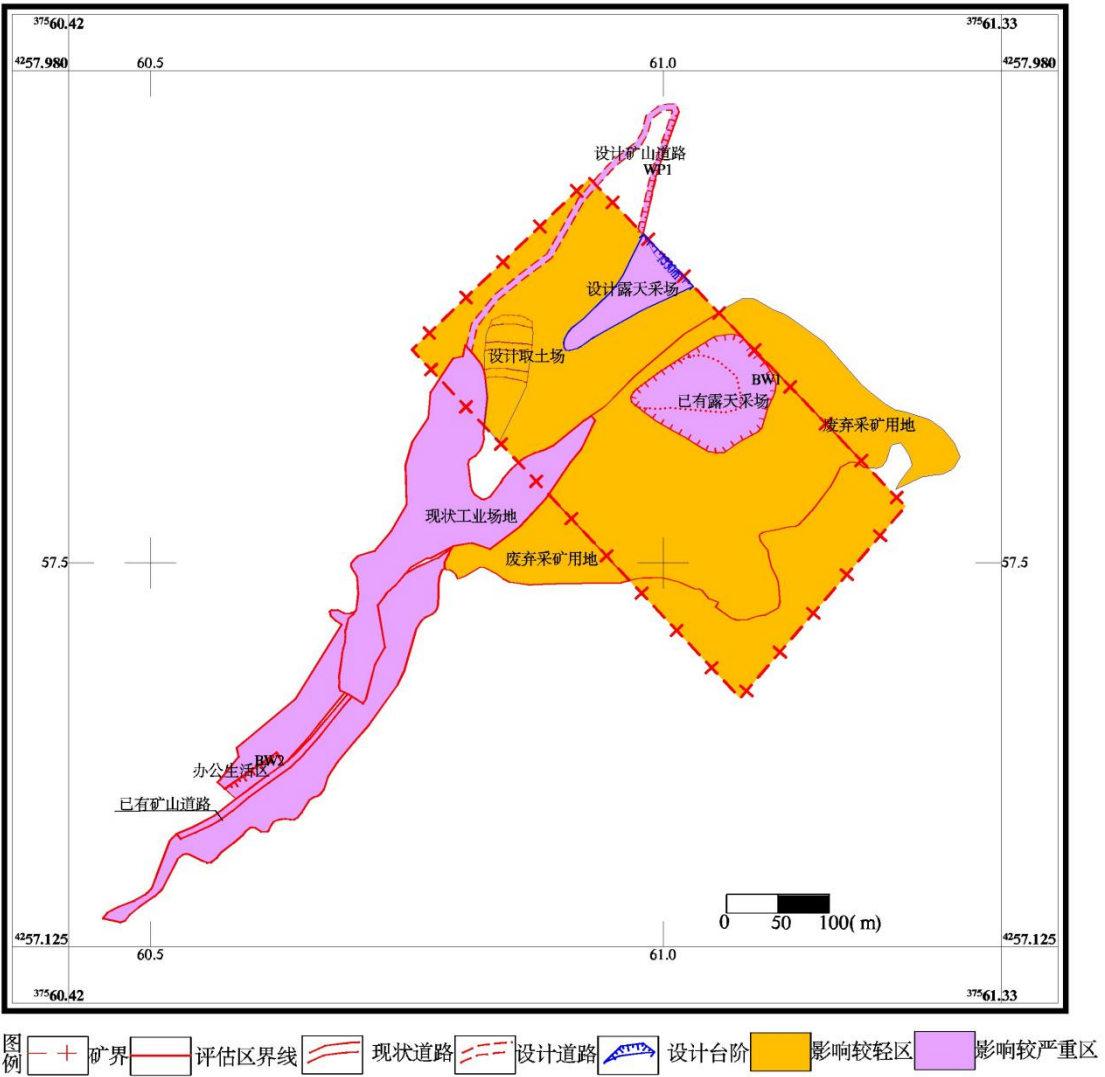
图 8-3-6 前五年矿山地质灾害危险性预测评估分区图
