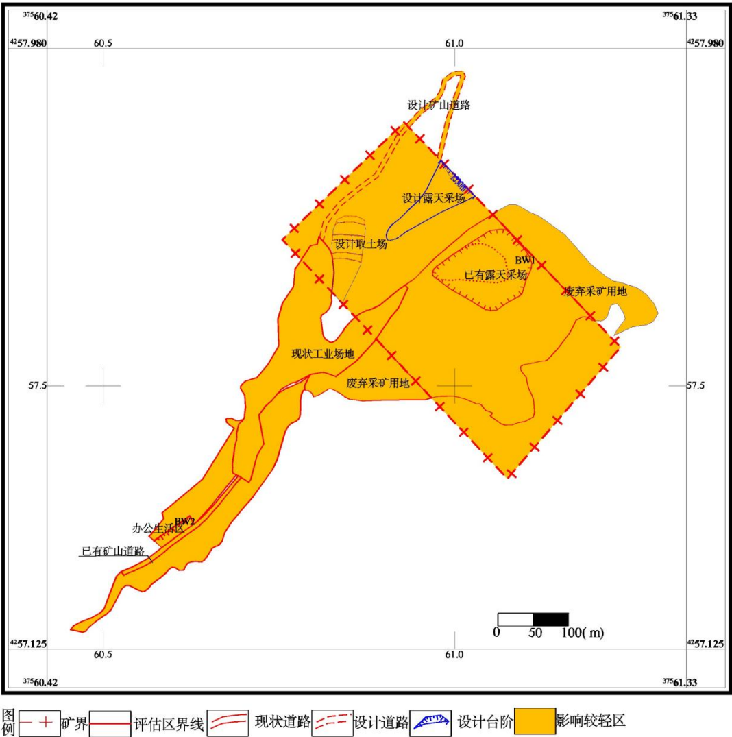
图8-3-8 五年期采矿活动对含水层影响与破坏预测评估分区图
