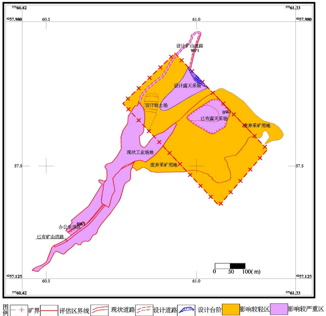
图 8-3-7 服务期矿山地质灾害危险性预测评估分区图
