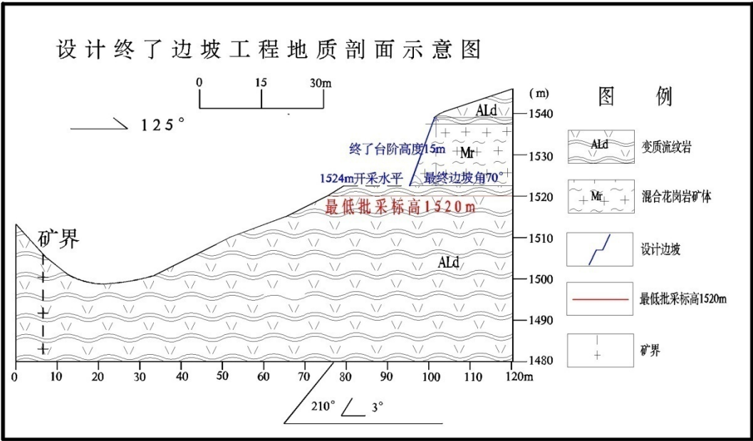
图 8-3-1 设计终了边坡剖面图
