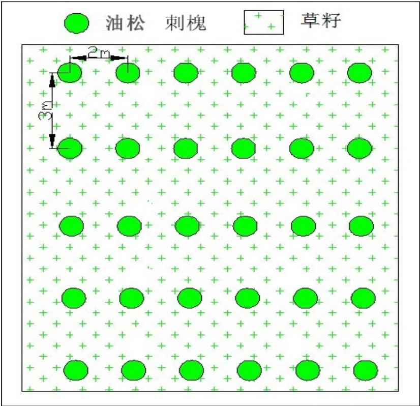
图 11-4-2 油松配置设计图
