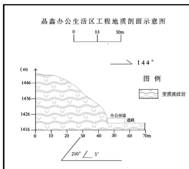
图 8-3-4 工业场地剖面示意图
