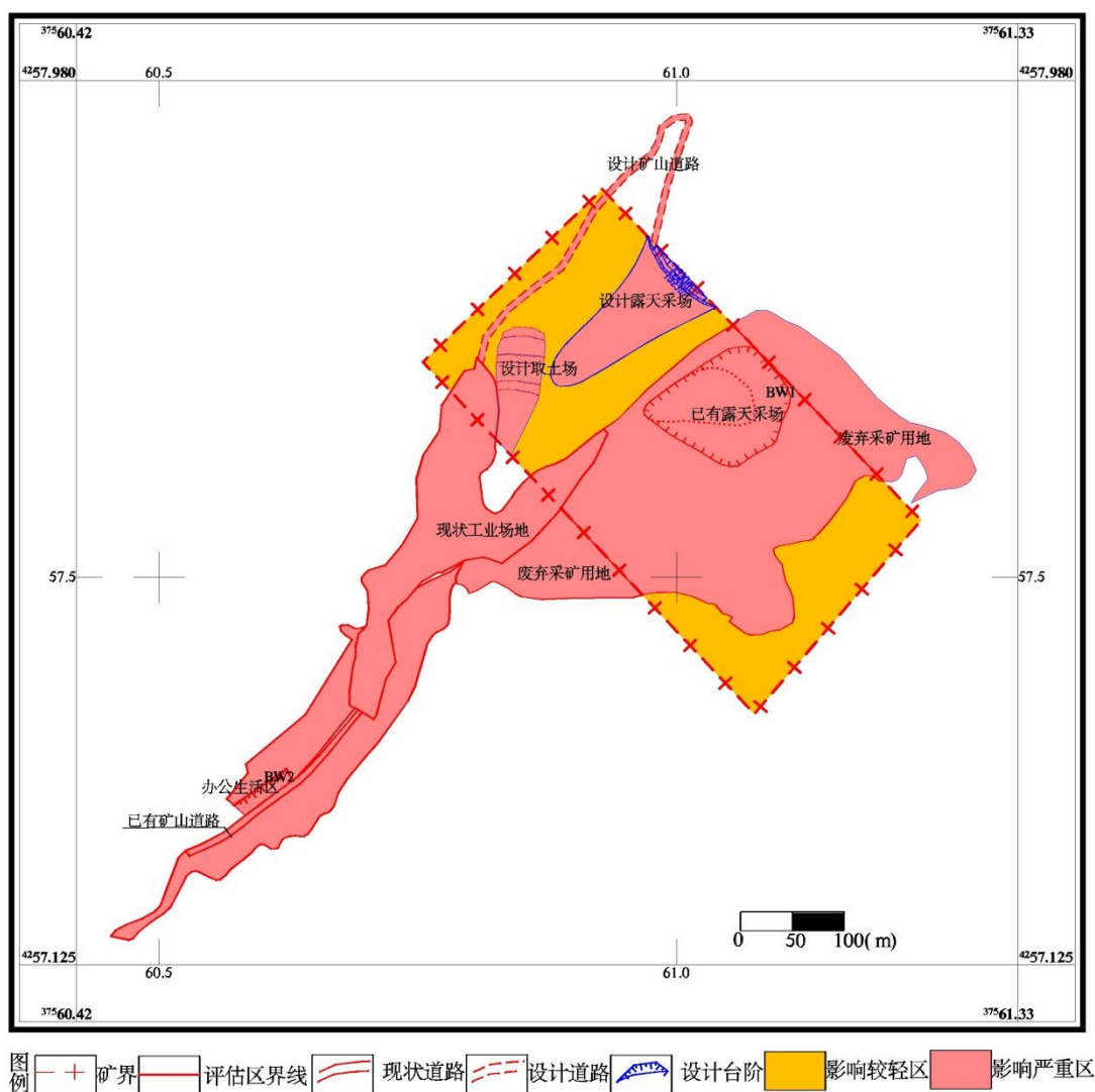
图 8-3-11 服务期采矿活动对地形地貌影响与破坏预测评估分区图
