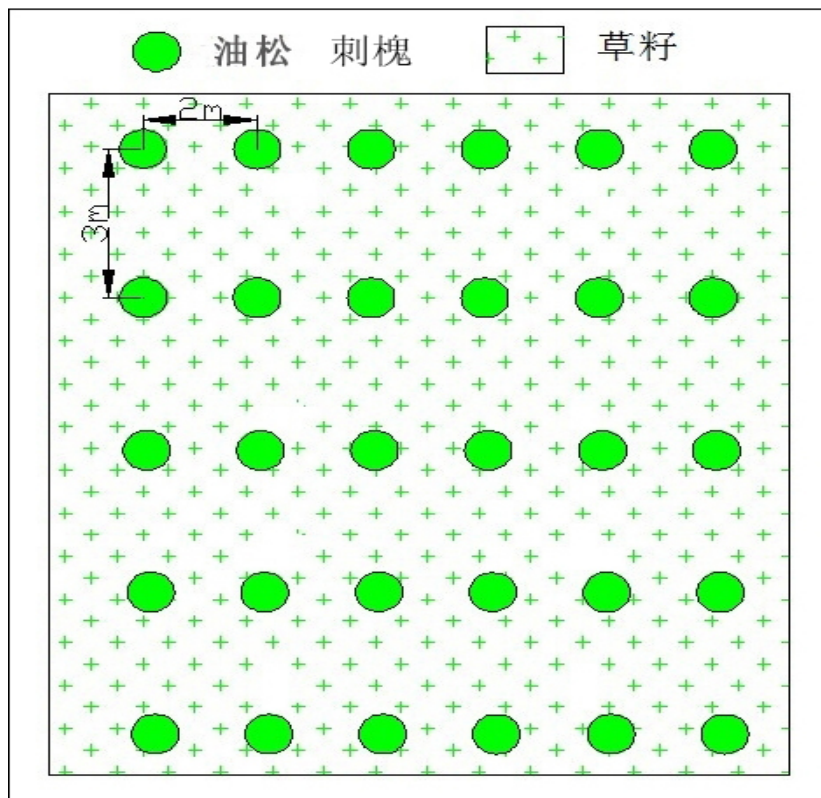
图 11-4-1 油松配置设计图
