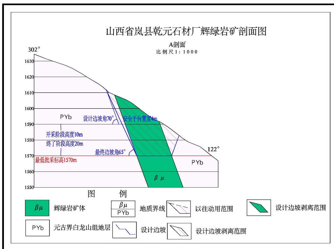
图 8-3-1 终了边坡剖面图
