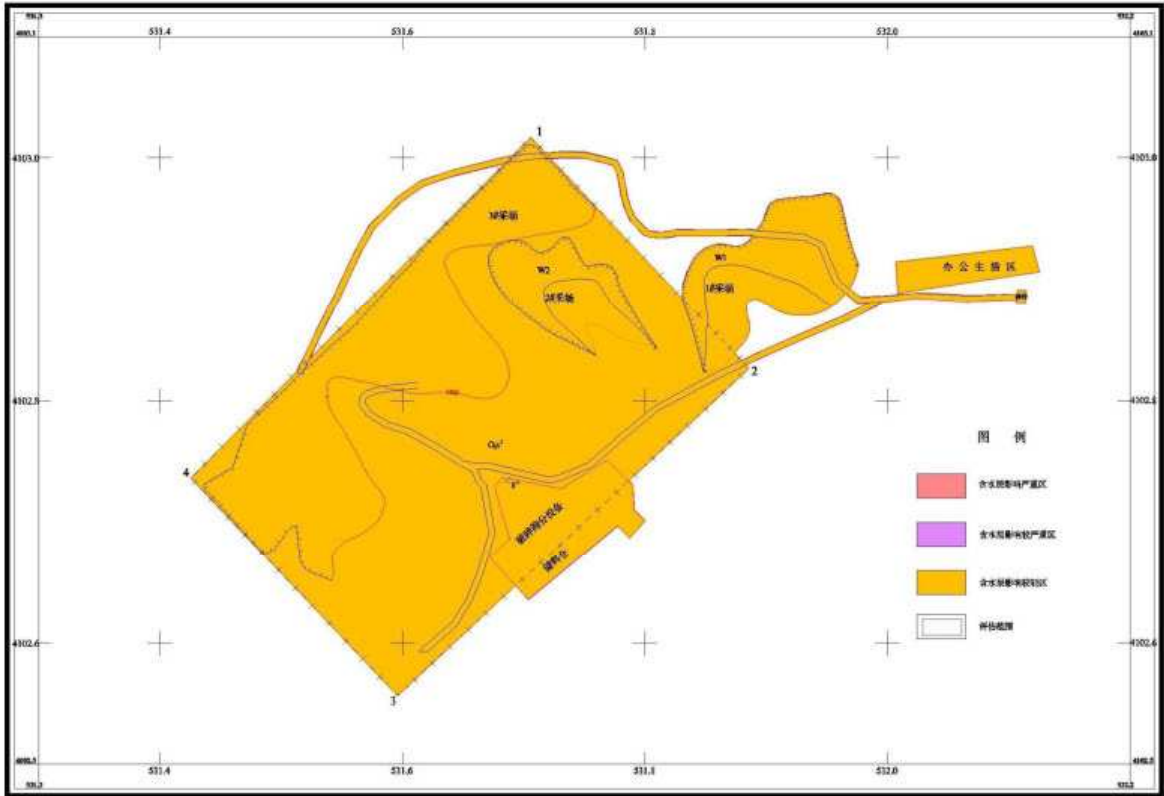
图 8-2-2 含水层现状评估图
