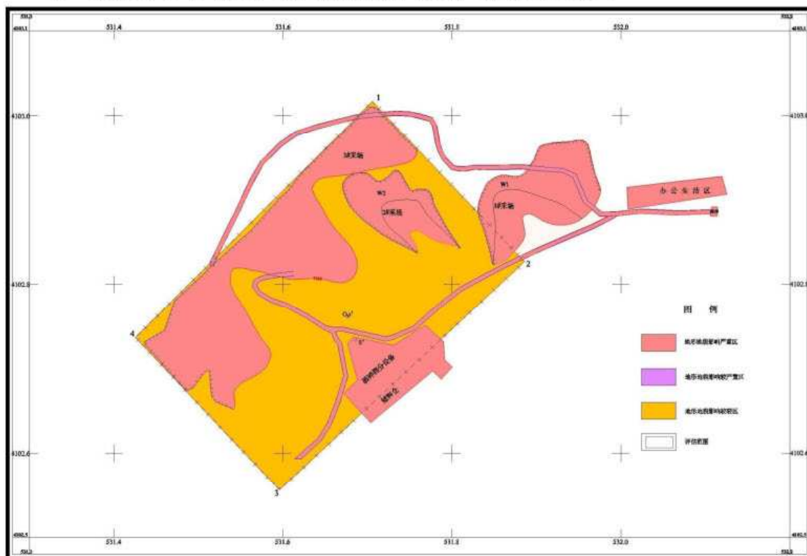
图 8-2-7 地形地貌现状评估图
