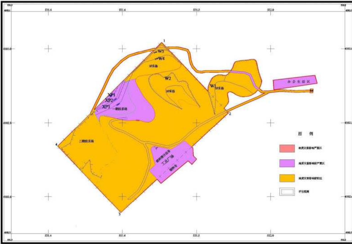
图 8-3-2 服务期地质灾害危险性预测评估分区图
