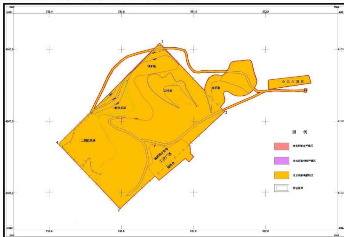
图 8-3-3 服务期采矿活动对含水层影响或破坏预测评估分区图
