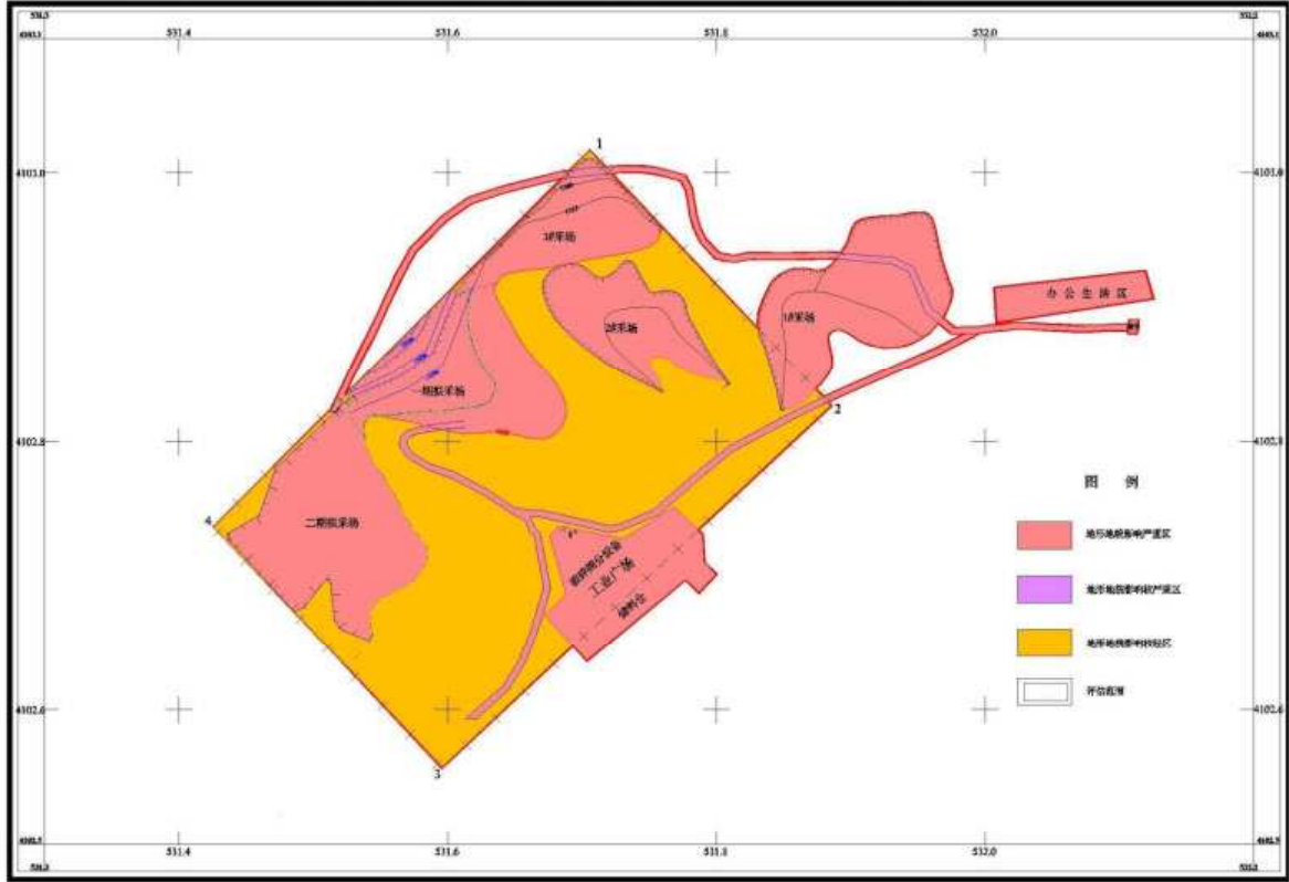
图 8-3-4 服务期采矿活动对地形地貌景观的影响与破坏预测评估分区图
