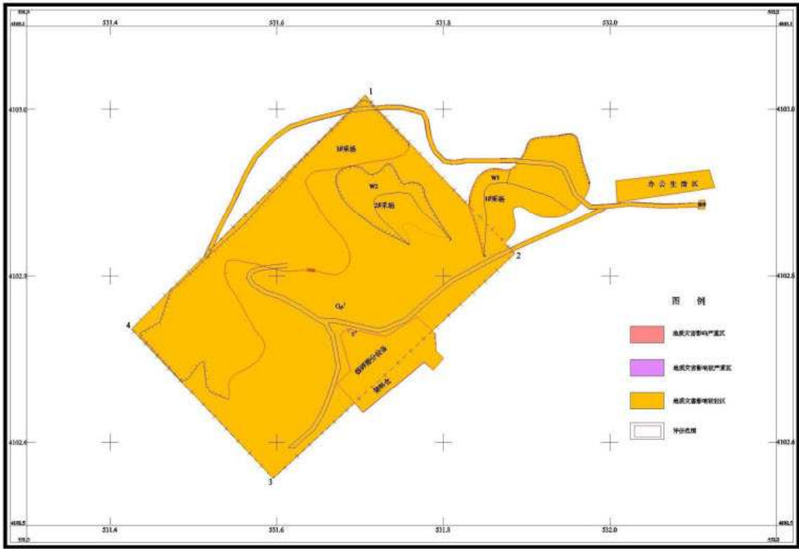
图 8-2-2 地质灾害现状评估图
